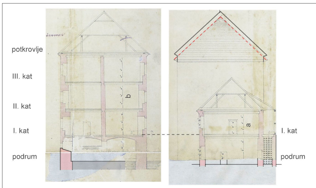
F. 98. 1873/76. kvadratna kula presjeci i pokušaj poravnivanja na nivou 1. kata (analiza B. Križanić 2025.)
