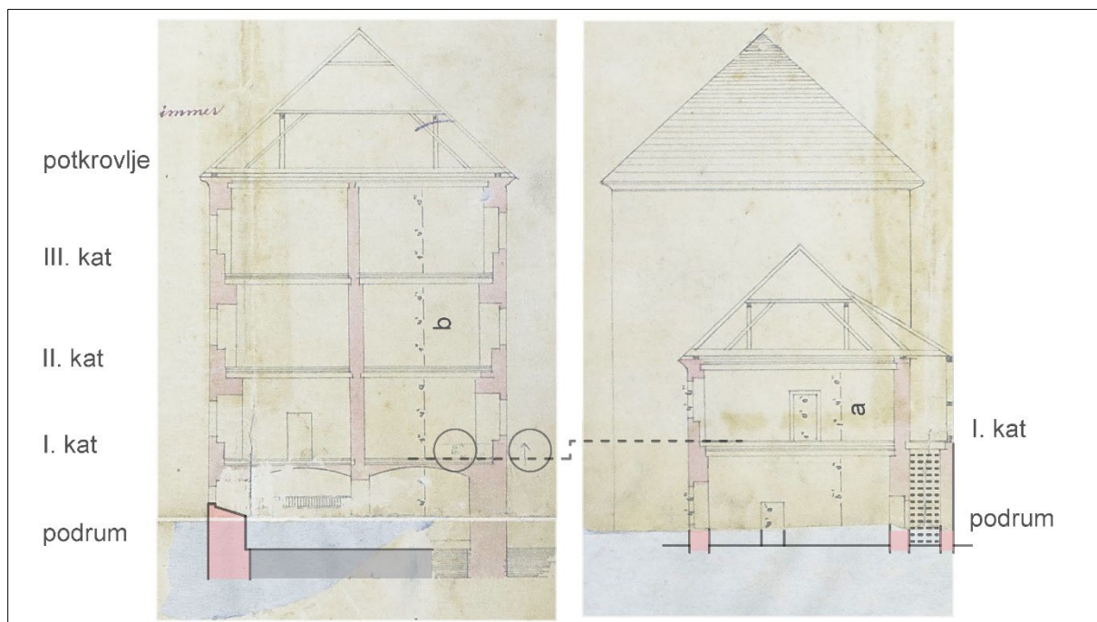
F. 1873/76. Kvadratna kula presjeci – izvorni nacrt i greške prikaza (analiza B. Križanić 2025.)
