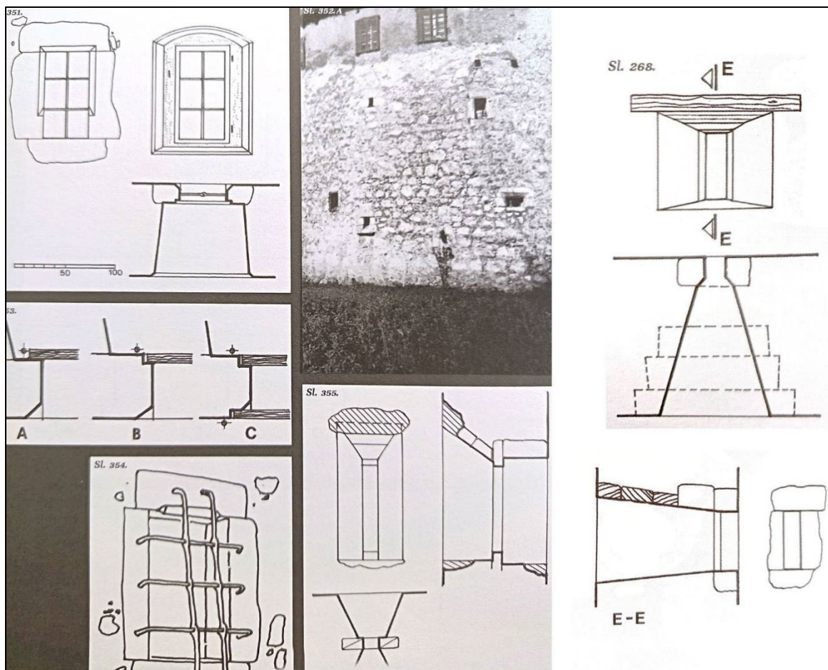
F. 102. Detalji prozora (Horvat, 2014)
