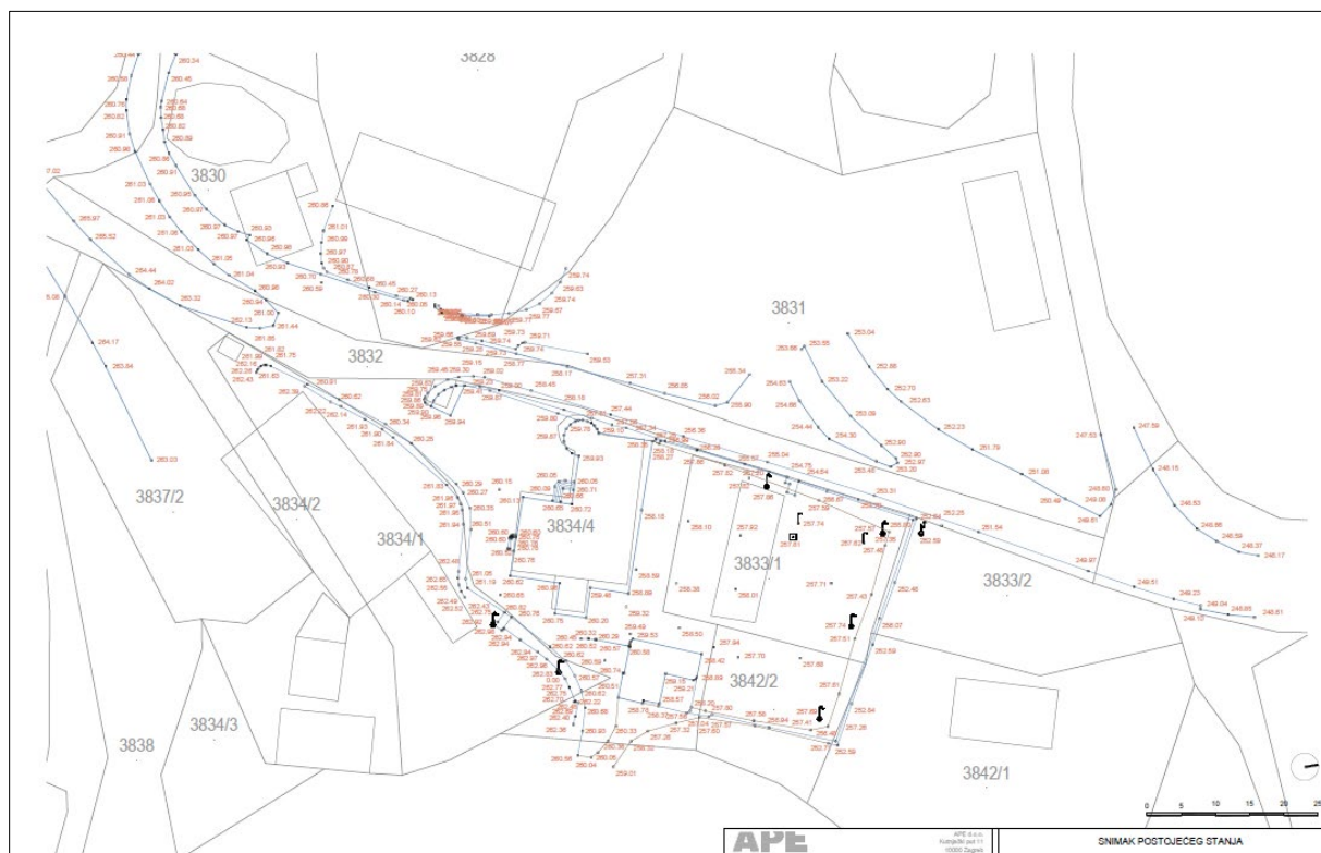
F.17. Geodetska snimka postojećeg stanja grada (Geokom d.o.o. 2025.)
