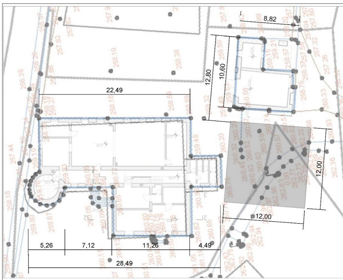
F. 101. Uklop arhitektonske snimke postojećeg stanja 2025. na geodetsku podlogu 2025. (analiza B. Križanić 2025.)
