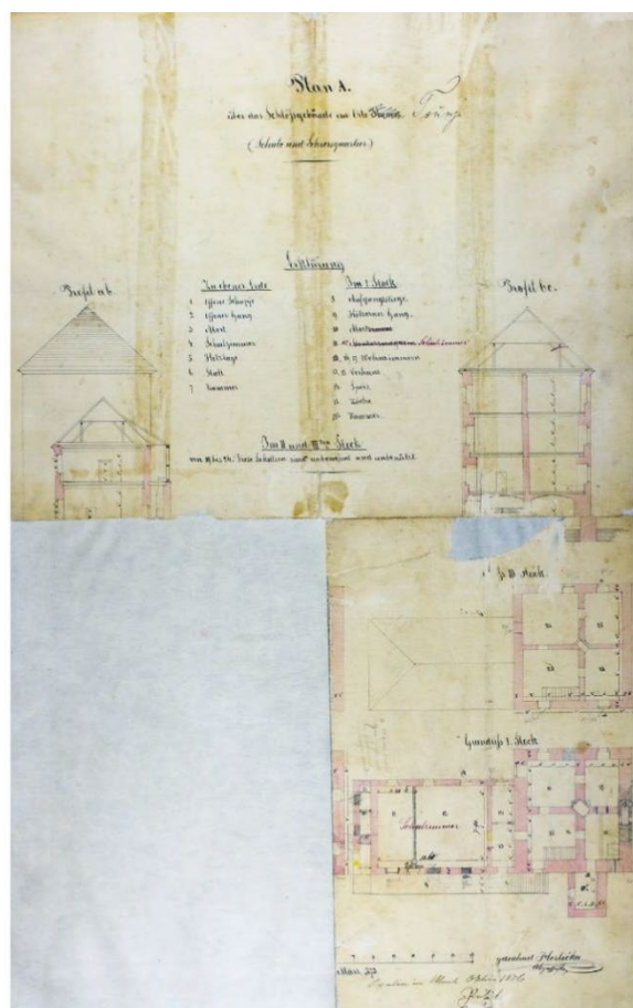
F. 72. PLAN A 1873. /76. – tlocrti 1. i 3. kata kule i zgrade uz kulu, presjeci kroz kulu i zgradu (DA-KA, Klc, oštećen izvorni, u boji)
