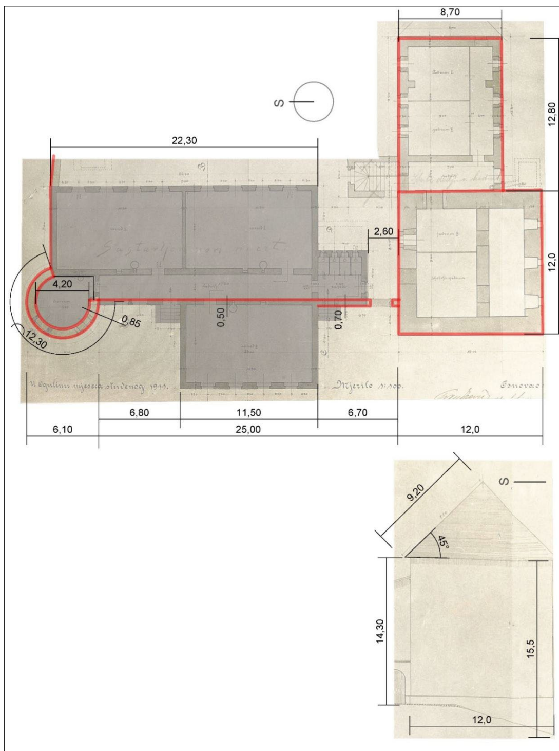
F.100. Nacrt interpolacije zgrade škole u strukturu grada - 1911.g. (metarski sustav) (analiza B. Križanić 2025.)
