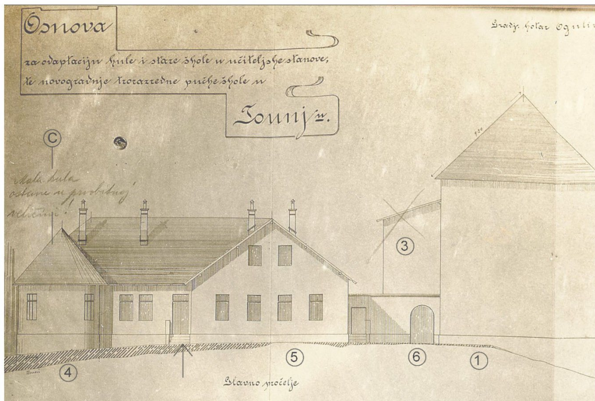
F. 78. Nacrt nove školske zgrade uz stari grad – gornji dio nacrtu – glavno (zapadno) pročelje ( inv. br. 7596 , foto Szabo, MKM-FKB)
