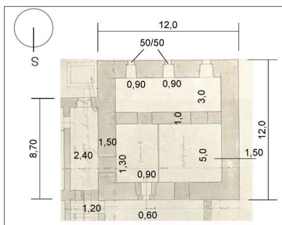
F. 97. 1911. Kvadratna kula tlocrti podruma – iz snimke post. stanja grada (analiza B. Križanić 2025.)
