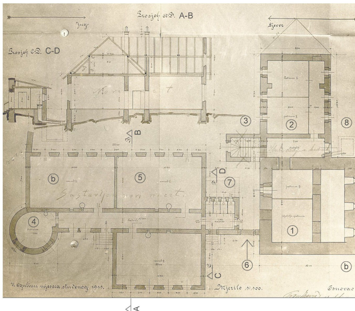
F.79. Nacrtna dokumentacija grada s novom školskom zgradom – donji dio nacrt, tlocrt, presjek ( inv. br. 7596 , foto Szabo, MKM-FKB)
