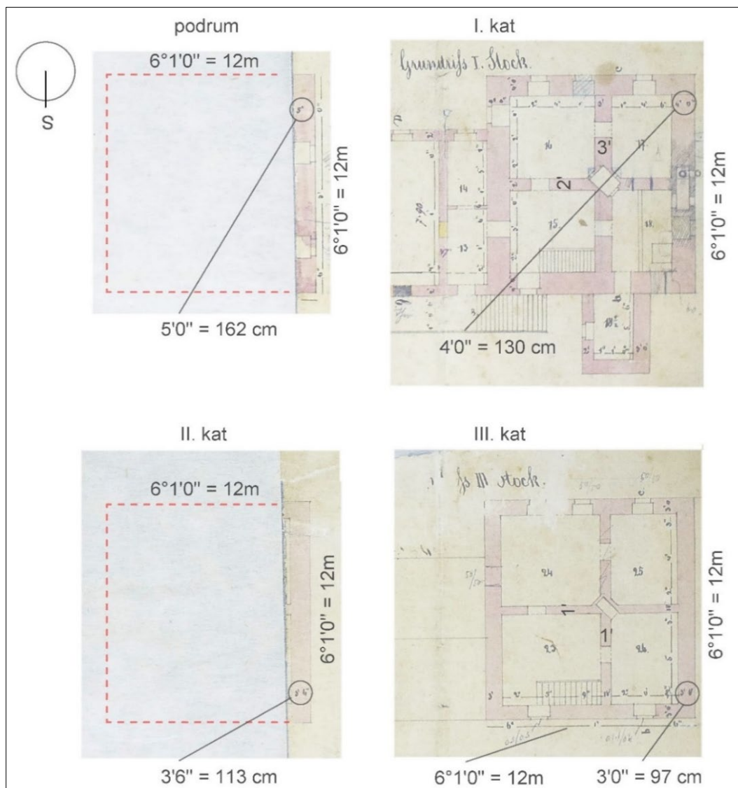
F. 96. 1873/76. Kvadratna kula tlocrti po etažama – iz originalnog nacrtu (analiza B. Križanić 2025.)
