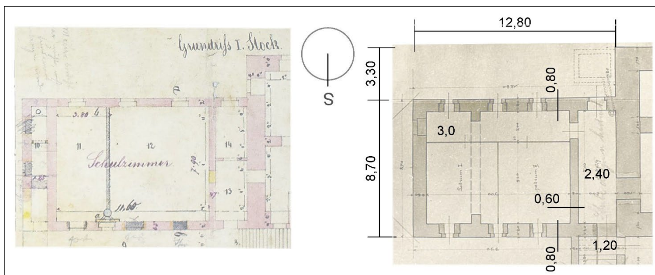
F.99. 1873/76. nacrt 1. kata i 1911. nacrt podruma zgrade uz kulu (hvati/metri) (analiza B. Križanić 2025.)
