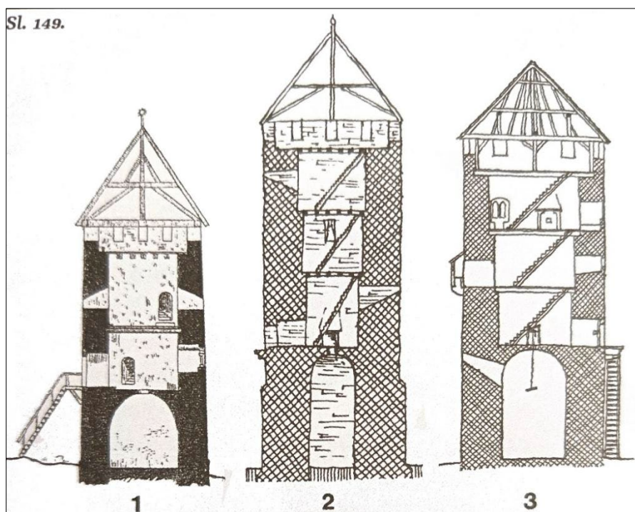
F. 116. Tipovi kula i krovšta s čardakom (braništem). 1.G. Szabo 2.O. Pipper 3.I. Villena (Z.Horvat, 149:2014.)
