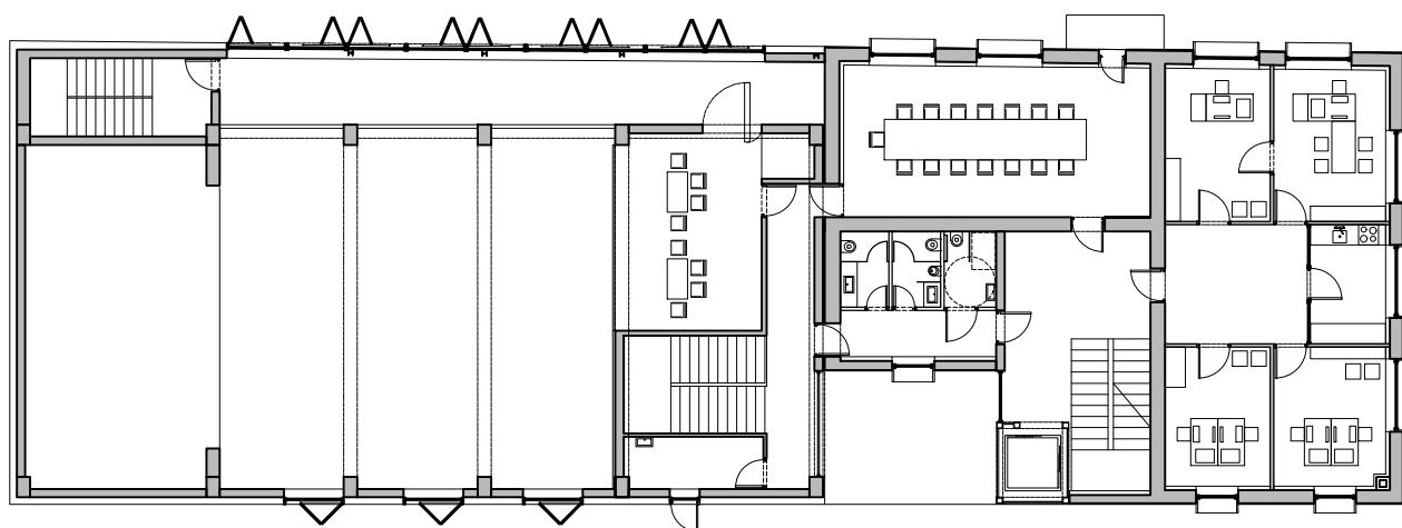
TLOCRT 1. KATA
