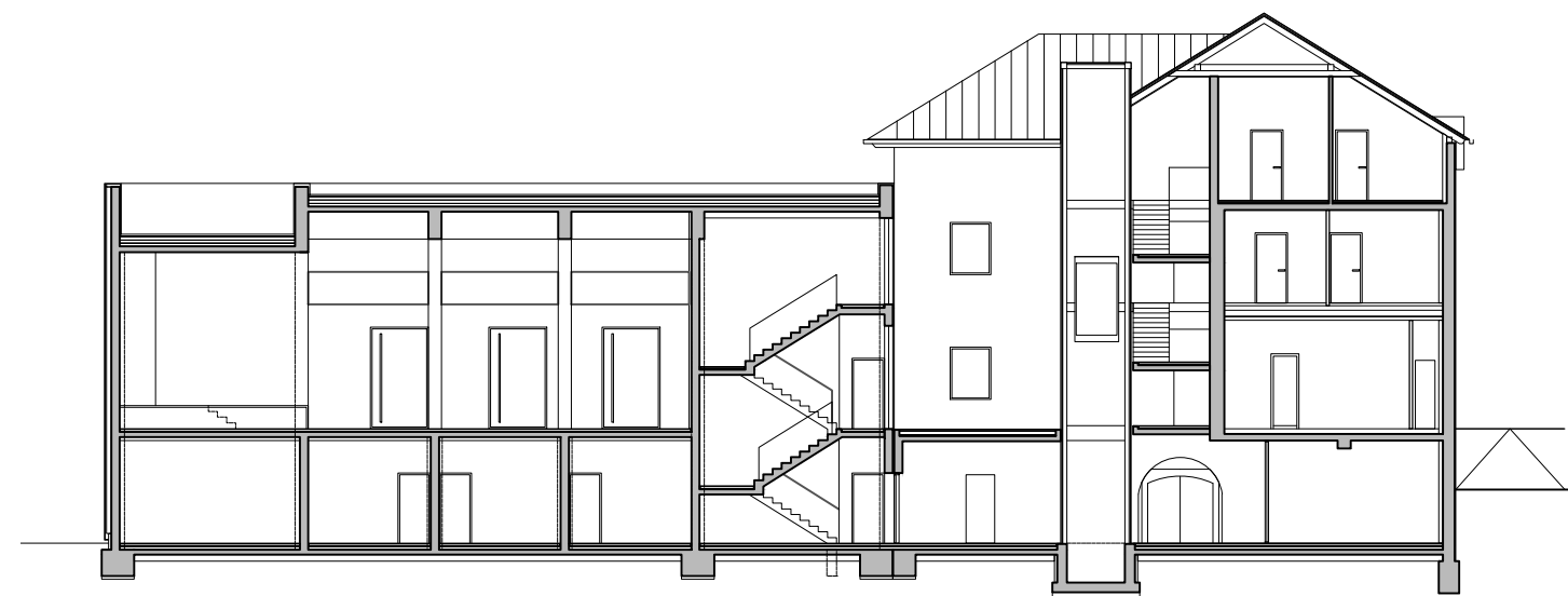
UZDUŽNI PRESJEK
