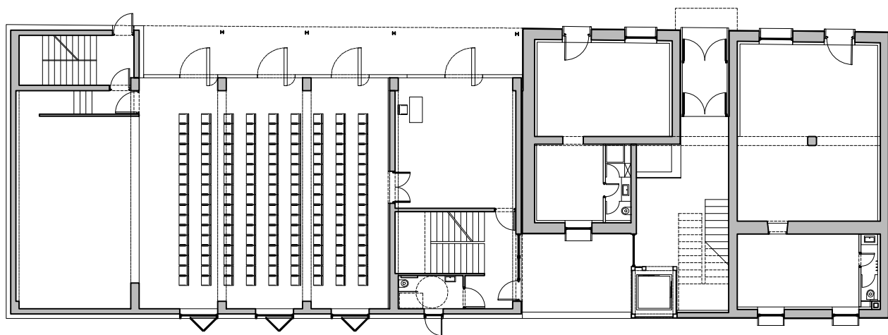
TLOCRT PRIZEMLJA
