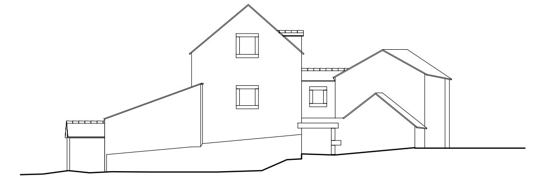
ZAPADNO PROČELJE
