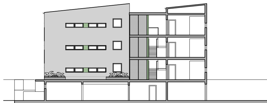
POPREČNI PRESJEK
