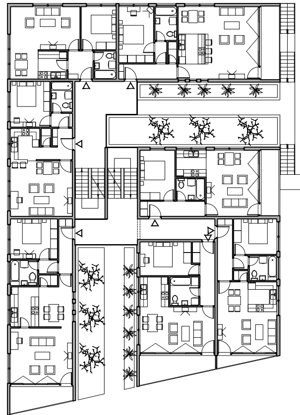
TLOCRT 2. KATA
