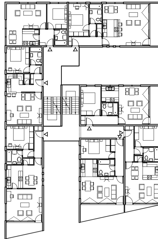
TLOCRT 3. KATA
