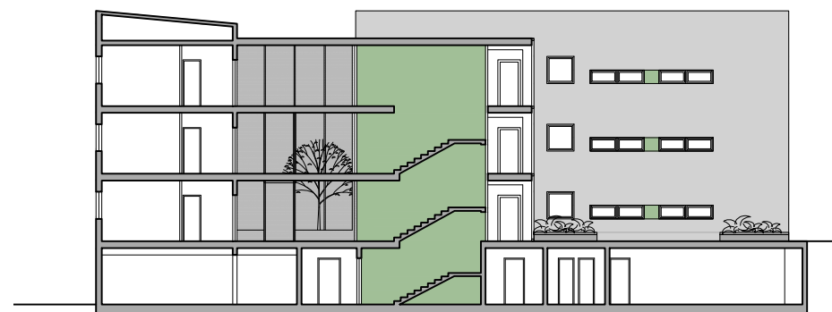
UZDUŽNI PRESJEK
